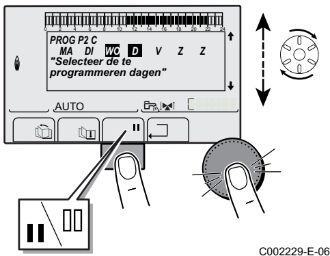
Afb.28 Een dag selecteren/deselecteren
